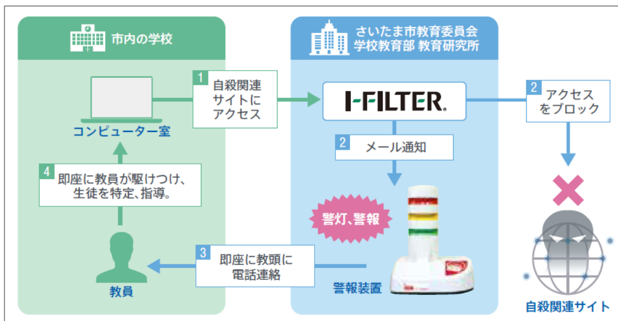
〈「i-FILTER」と警報装置の連動イメージ〉
